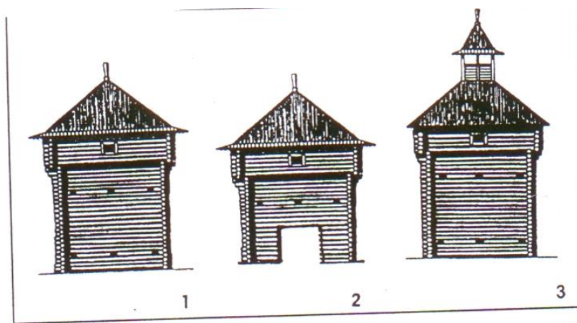
Рис. 5. Разновидности деревянных башен сибирских острогов (по Н.П. 1 — угловая башня; 2 — проездная башня; 3 — сторожевая башня с караульной вышкой)
