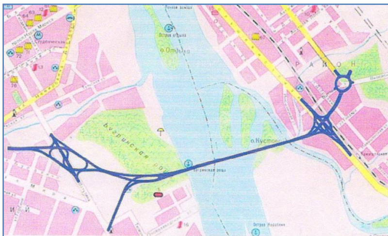
Схема расположения будущего третьего моста через Обь.
