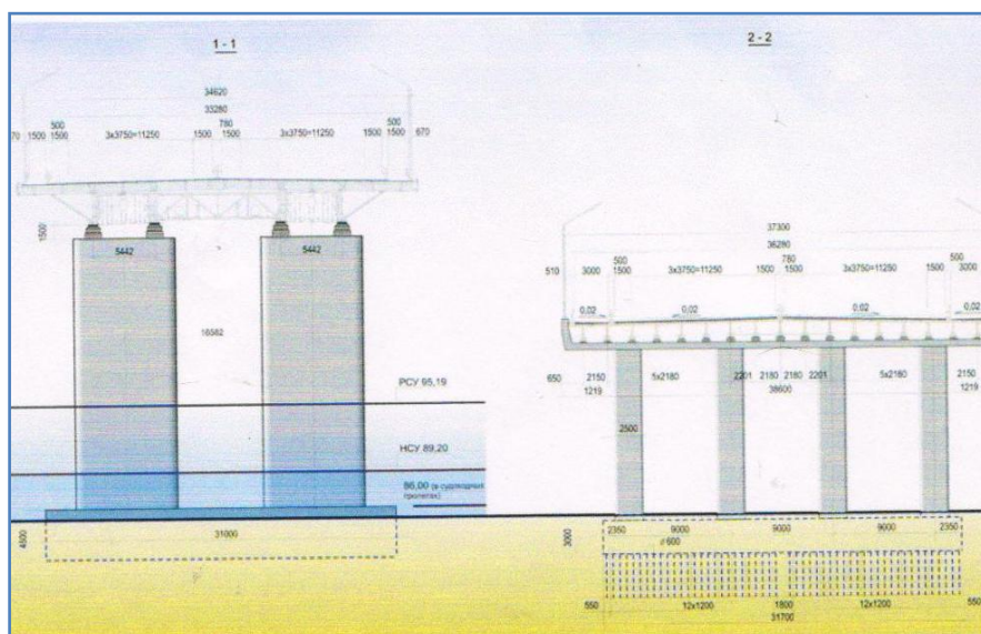
Поперечник третьего моста.
